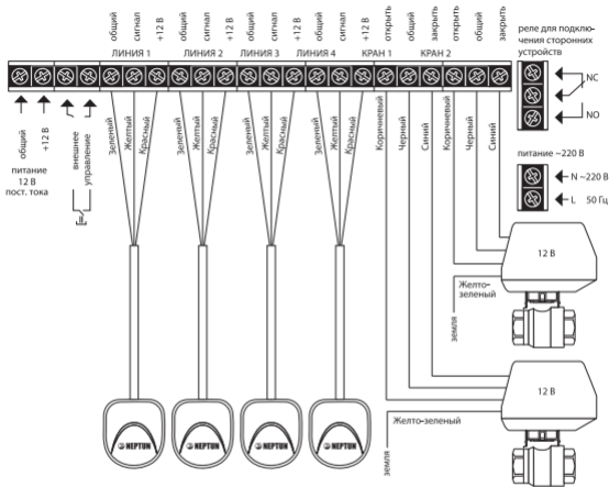
Рис. 4. Схема подключения кранов шаровых с электроприводом DePaLa 12 В к модулю управления Neptun ProW
